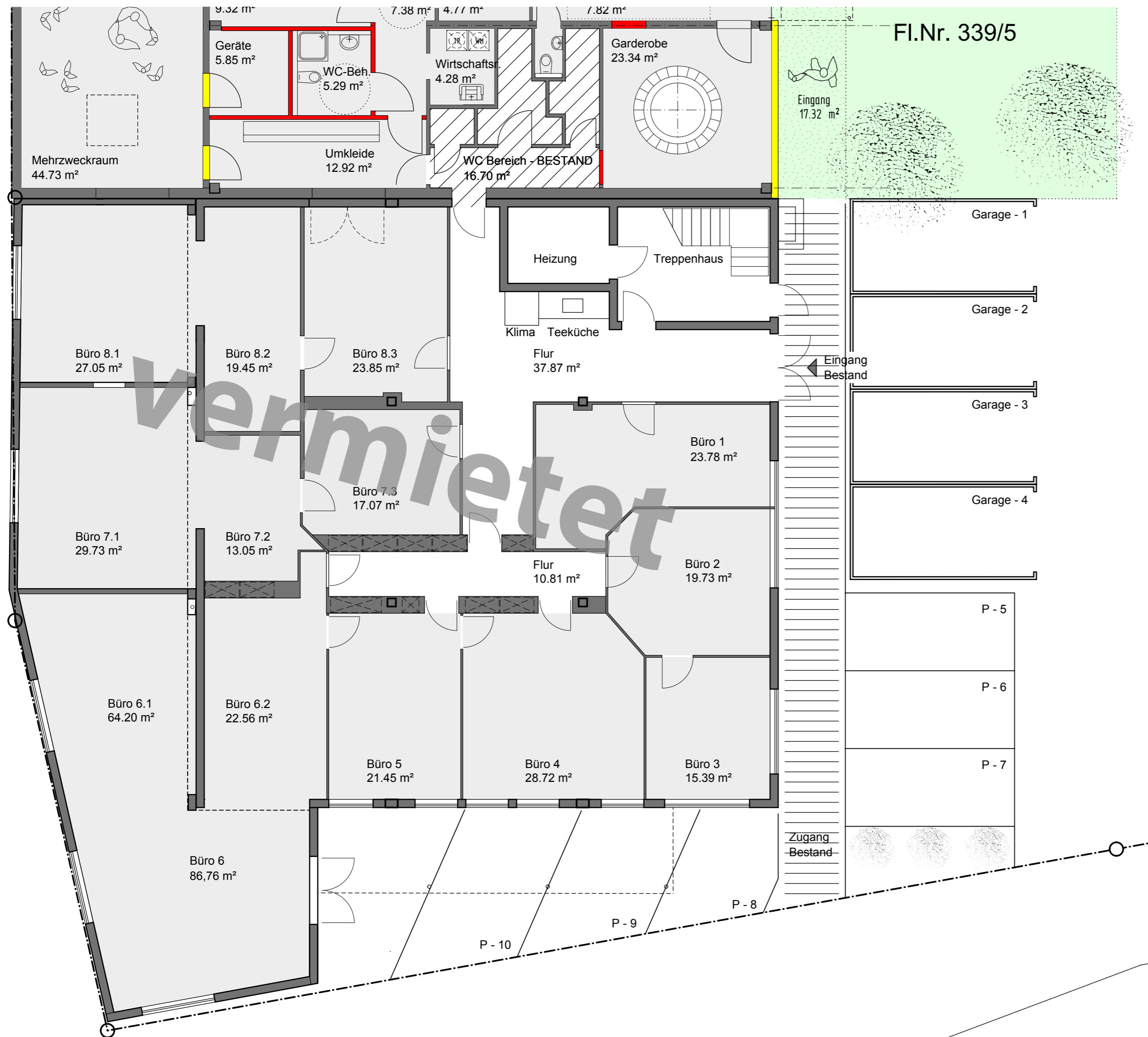
Grundriss Erdgeschoss
